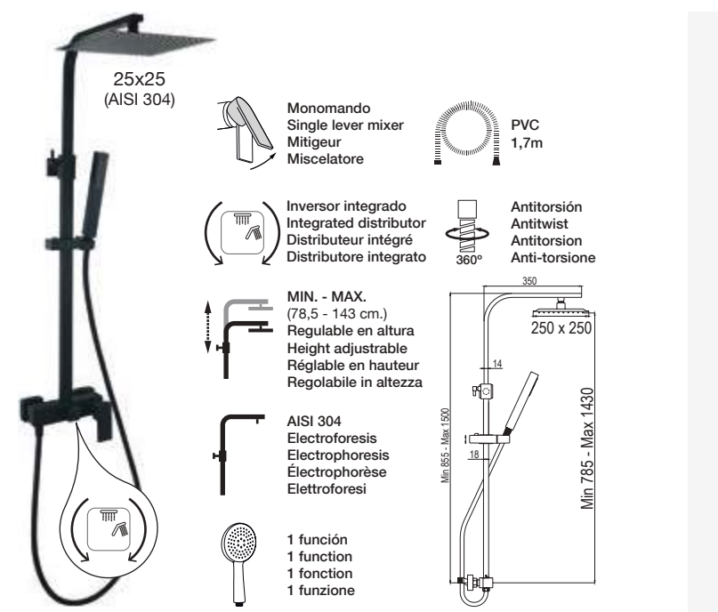
25x25 (AISI 304) Monomando Single lever mixer Mitigeur Miscelatore Inversor integrado Integrated distributor Distributeur intégré Distributore integrato MIN. - MAX. (78,5 - 143 cm.) Regulable en altura Height adjustable Réglable en hauteur Regolabile in altezza AISI 304 Electroforesis Electrophoresis Electrophorèse Elettroforesi 1 función 1 function 1 fonction 1 funzione PVC 1,7m Antitorsión Antitwist Antitorsion Anti-torsione 360° 350 250 x 250 Min 855 - Max 1500 Min 785 - Max 1430
