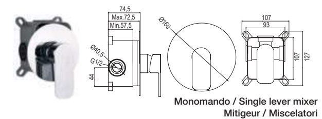
01VE2350CR 1 vía / 1 way / 1 voie / 1 via
