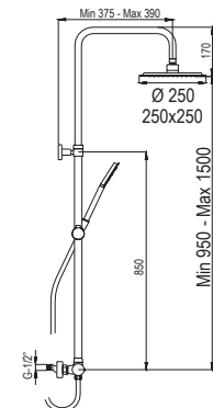
AISI 304 Tubo cromado Chrome tube Barre chromé Barra cromata
