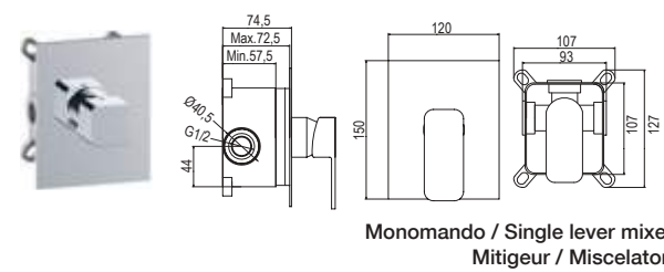
01QBE350CR 1 vía / 1 way / 1 voie / 1 via
